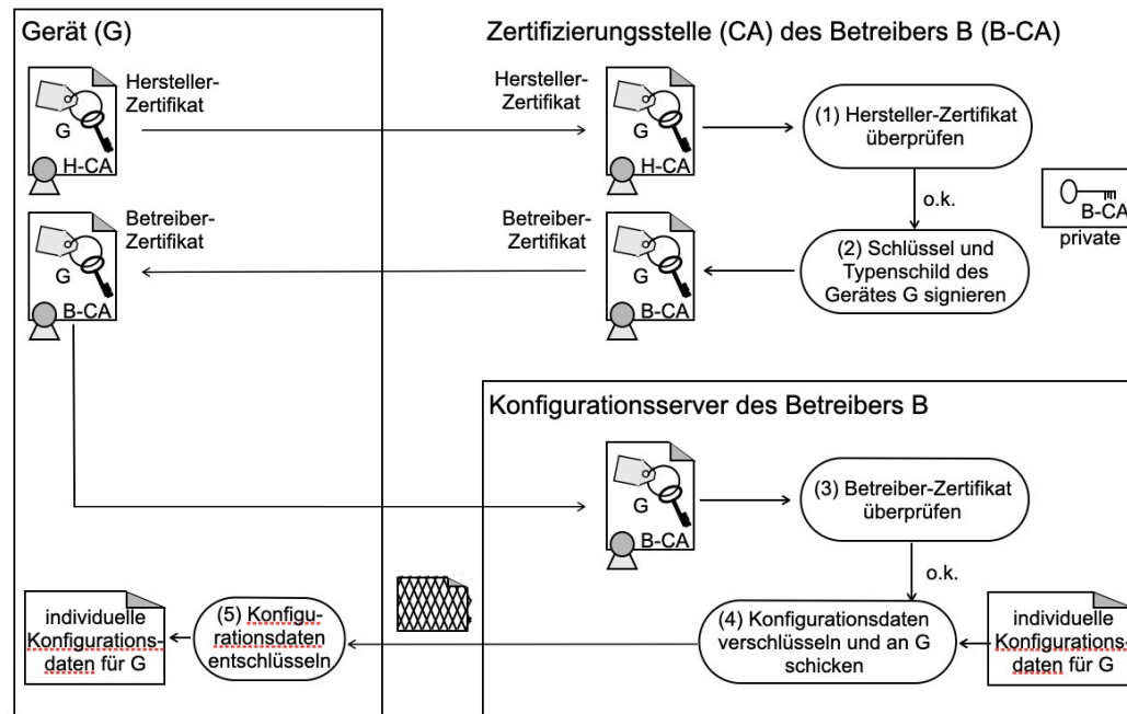
(b) Ablauf im Netz des Betreibers B
